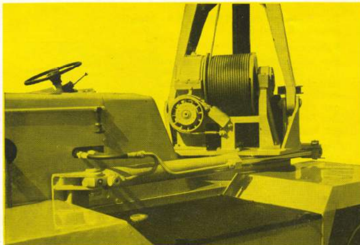
Das Hub- und Drehwerk des AK 50 B. Die Drehbewegung des um 80° schwenkbaren Auslegers erfolgt durch eine doppelt wirkende Einkolbenpresse. Das zweistufige Hubwerk wird hydraulisch betätigt, wobei die angeschlossene Hubwerksbremse automatisch arbeitet.
