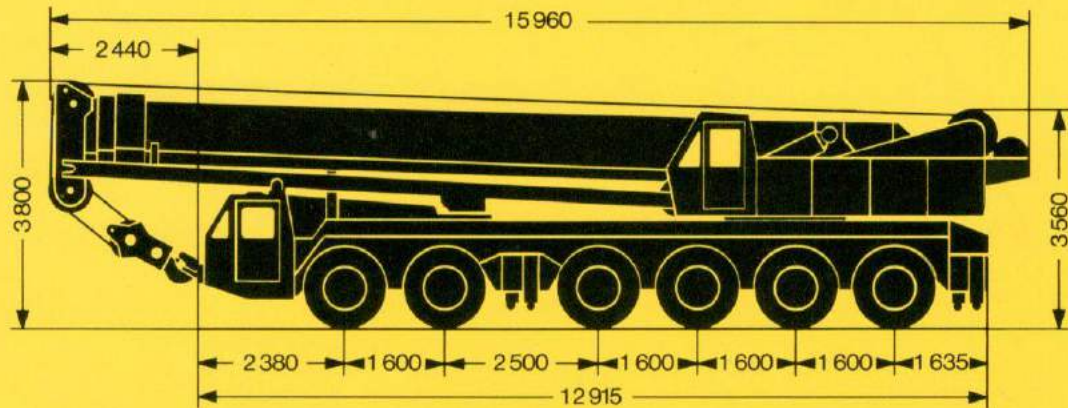
Die Achslasten (t). Kran in Fahrtstellung.
