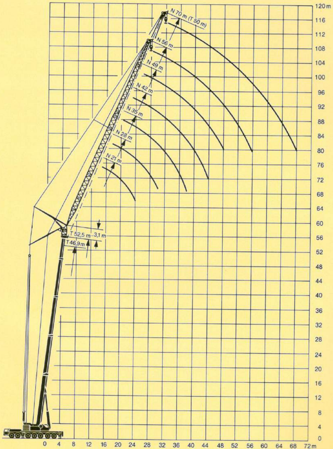
Teleskopausleger / Telescopic boom / Flèche télescopique: 83°
